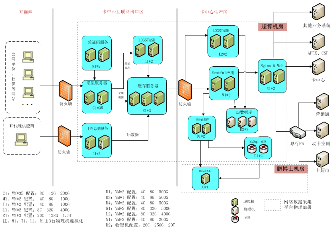
网络数据采集平台物理部署图
